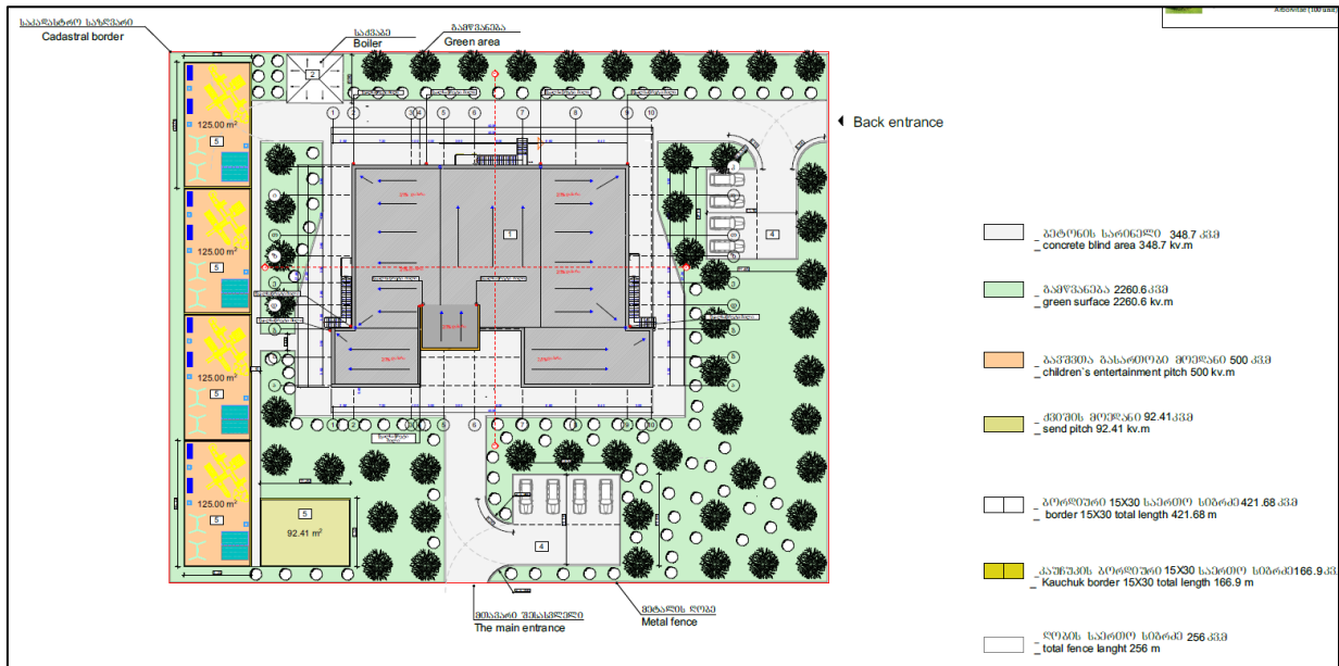
გამოსახულება 3. გენ. გეგმა
