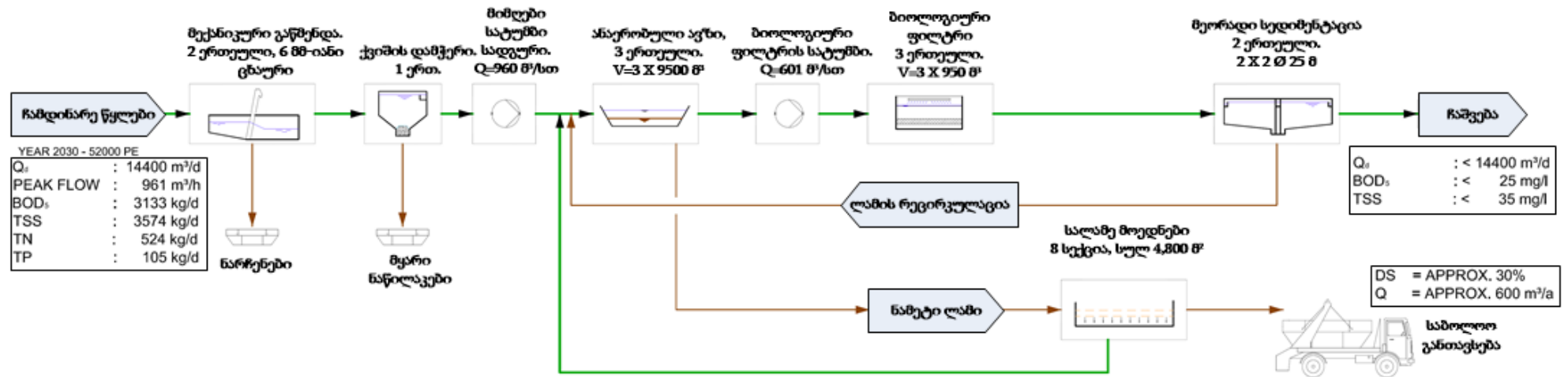
ნახაზი 4.3.1. ჩამდინარე წყლების გაწმენდის ტექნოლოგიური სქემა - ფაზა 1.
