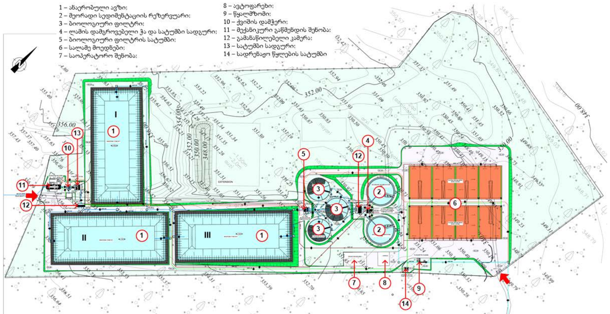
ნახაზი 4.2.1. საპროექტო გამწმენდი ნაგებობის გენ-გეგმა, 1:500
