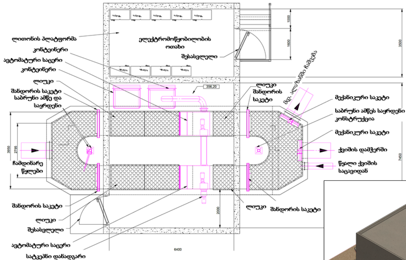
მექანიკური გაწმენდის შენობის გეგმა (მ 1:50) და 3D გამოსახულება
